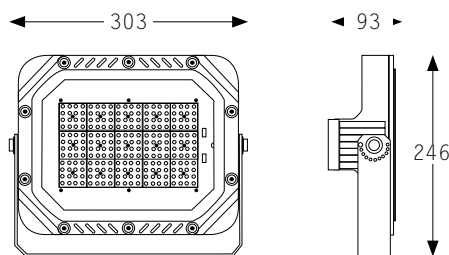
Disegno Tecnico
