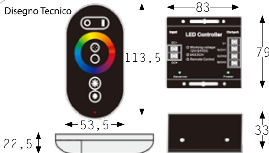
Disegno Tecnico
