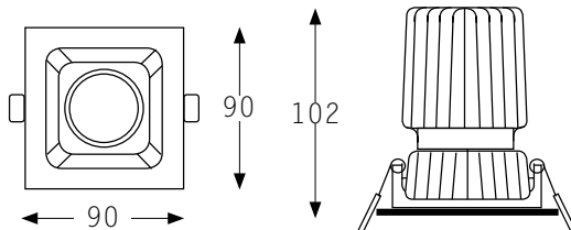
Disegno Tecnico
