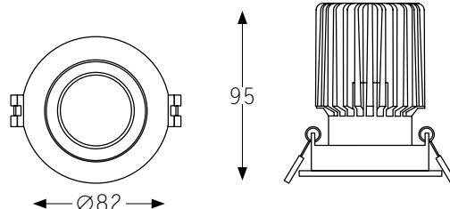
Disegno Tecnico
