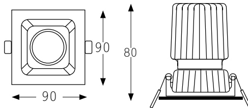
Disegno Tecnico
