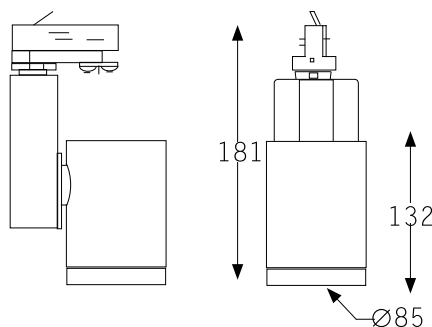
Disegno Tecnico
